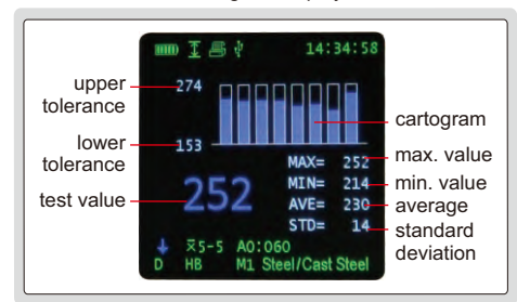
histogram display
